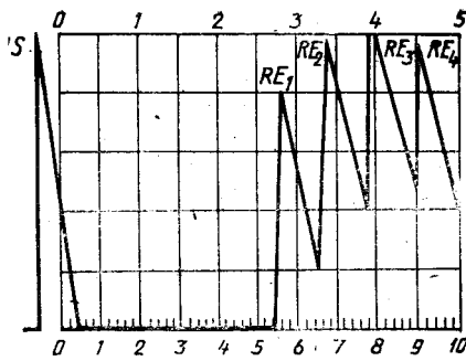
Установление звукового сигнала при помощи преобразователя с двойными кристаллами
