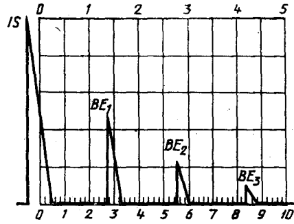
Удовлетворительное соединение
