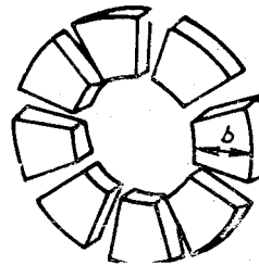
Блок упорных сегментов
