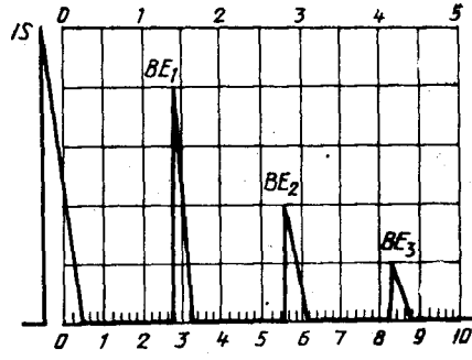
Плохое соединение
