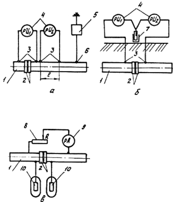
Рис. 34. Схемы включения измерительных приборов и устройств при опробовании и наладке изолирующих фланцев трубопровода: а - измерение сопротивления; б - определение эффективности действия; в - измерение и регулирование тока в шунтирующем резисторе; 1 - трубопровод; 2 - изолирующие фланцы; 3 - контакт с трубопроводом; 4 - многопредельный вольтметр; 5 - установка катодной защиты; 6 - точка дренажа; 7 - неполяризуемый медно-сульфатный электрод сравнения; 8 - регулировочный резистор; 9 - амперметр; 10 - токоотвод-протектор
