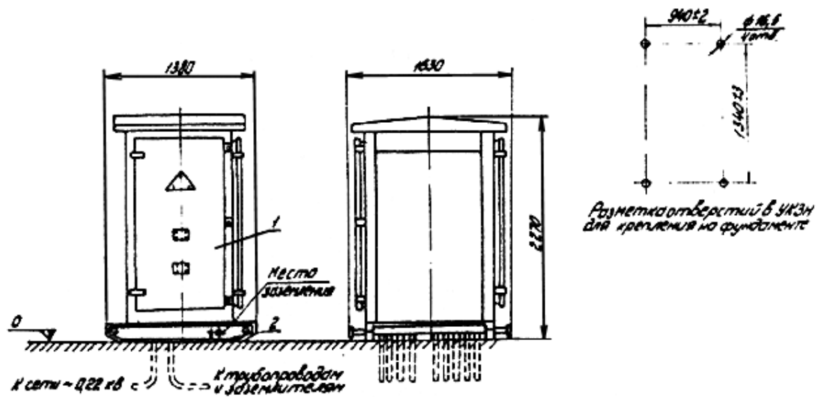
Рис. 1. Общий вид смонтированного устройства катодной защиты низковольтного УКЗН: 1 - блок катодных станций; 2 - салазки
