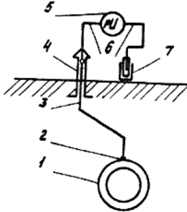
Рис. 31. Схема измерений разности потенциалов "труба -земля": 1 - трубопровод, 2 - контакт с трубопроводом; 3 - катодный вывод; 4 - контрольно-измерительный пункт; 5 - многопредельный вольтметр; 6 - измерительные провода; 7 - неполяризующийся медно-сульфатный электрод
