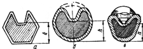
Рис.28. Измерение остаточной толщины в месте опрессовки: а - многогранное обжатие с жестким вдавливанием; б - местное вдавливание лункой; в - местное вдавливание ступенчатым опрессованием
