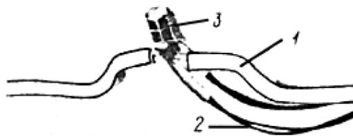
Рис. 29. Узел контактного соединения при монтаже анодных заземлителей:
